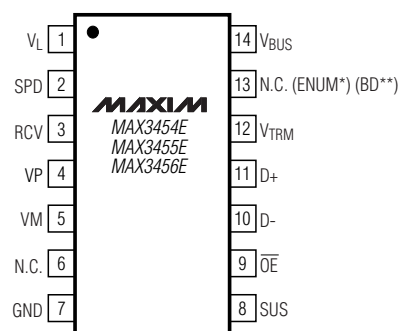
TSSOP
