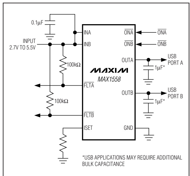
图 1. 典型应用电路
