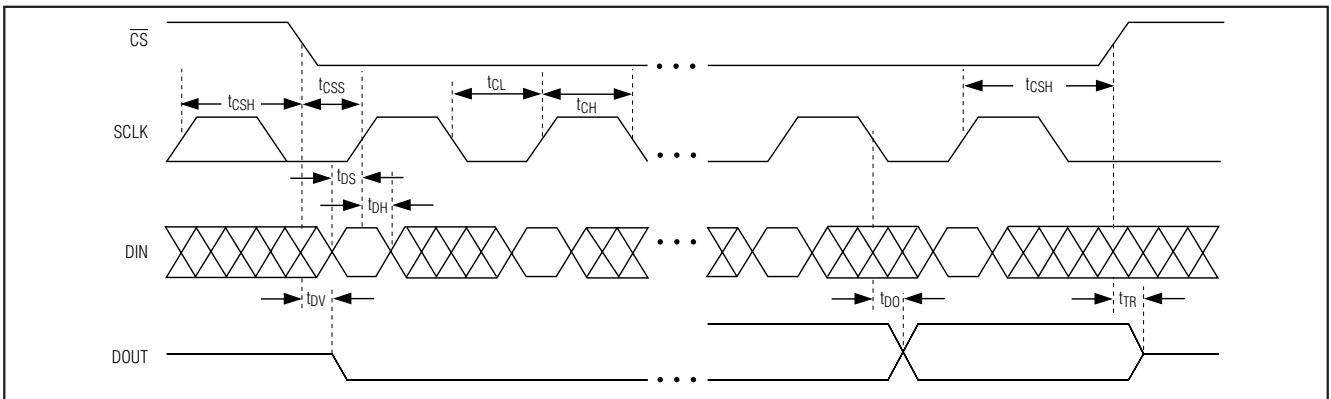
图 8. 详细时序图
