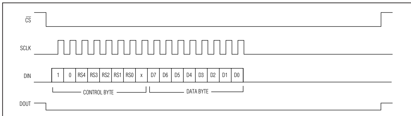
图 10. 串口 8 位写时序图
