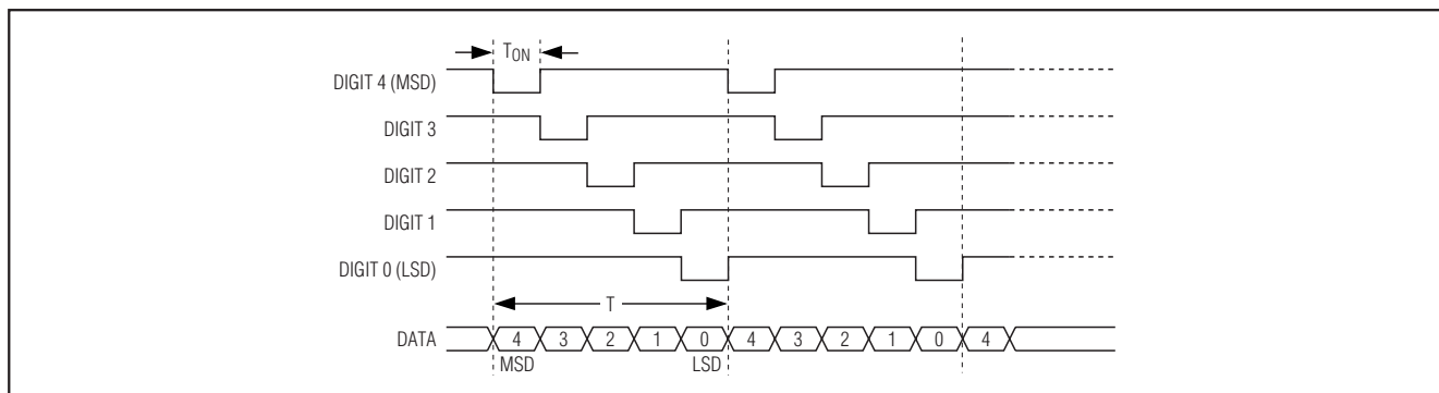
图 6. LED 电压波形——MAX1499
