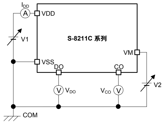
图6 测定电路2
