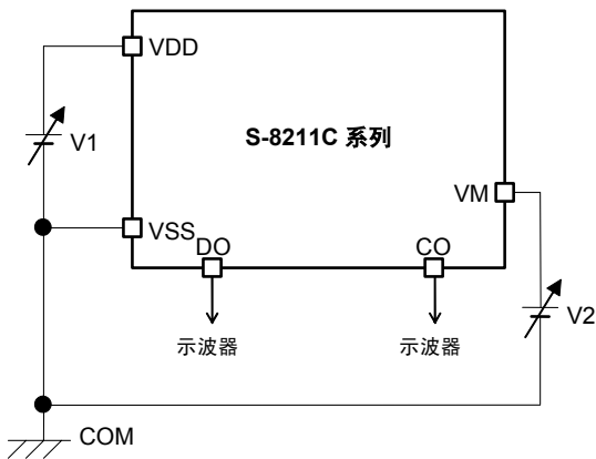
图9 测定电路5
