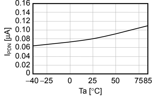
(2) I_{PDN}-T_a
