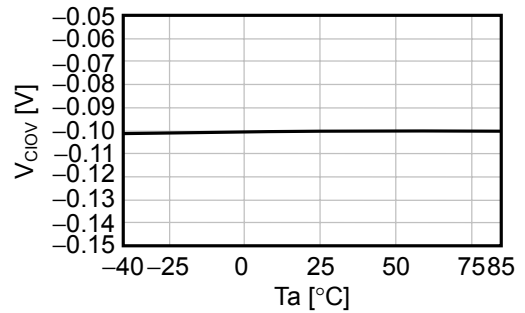
(12) V_{CIOV} - T_a
