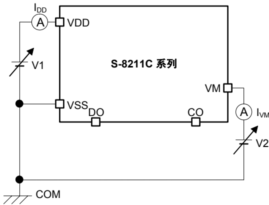
图7 测定电路3
