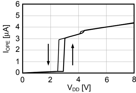
(3) I_{OPE}-V_{DD}
