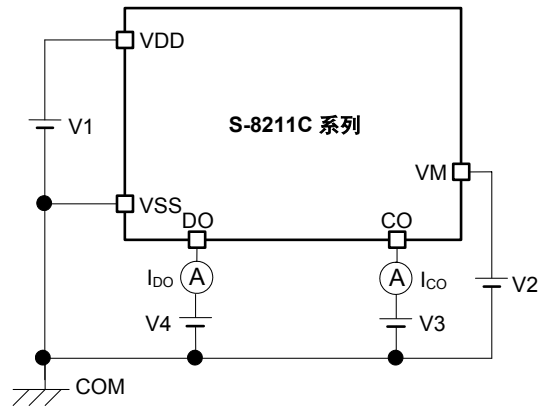
图8 测定电路4
