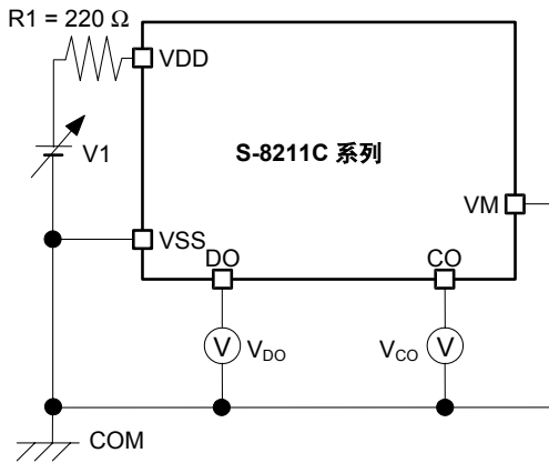
图5 测定电路1
