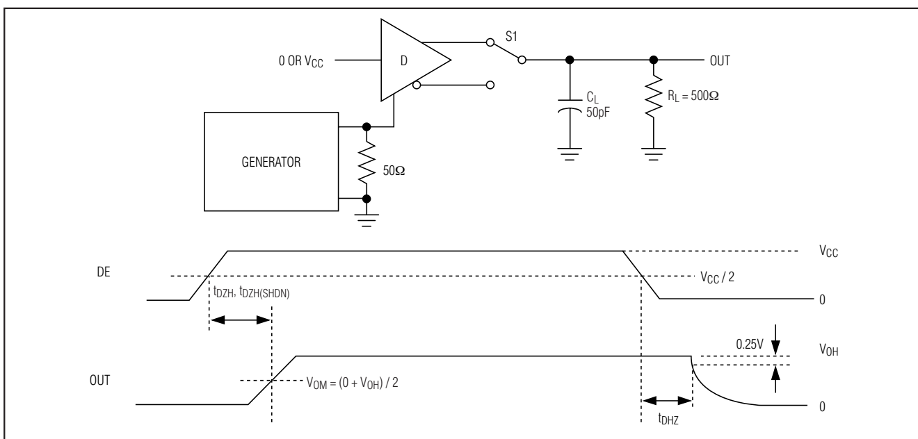
图4. 驱动器使能和禁用时序 ( t_{DZH} 、 t_{DZL} 、 t_{DZL(SHDN)} )
