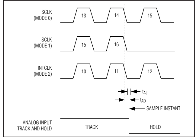
图21. 孔径时序图
