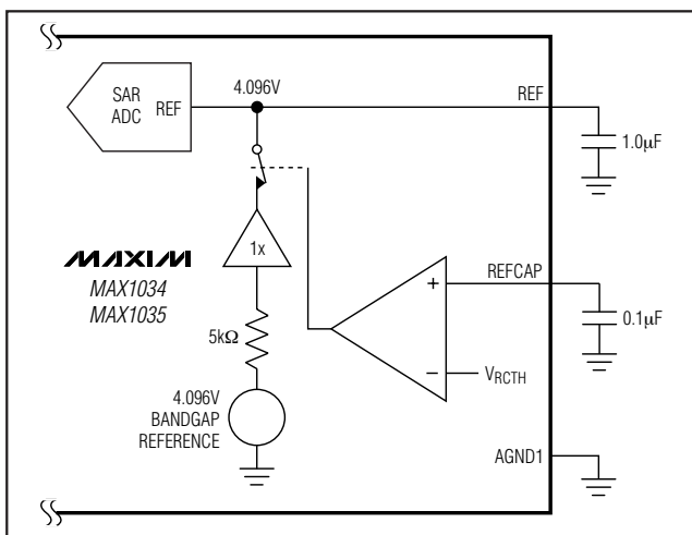
图17. 内部基准
