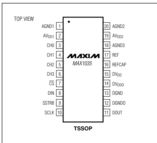
引脚配置 (续)
