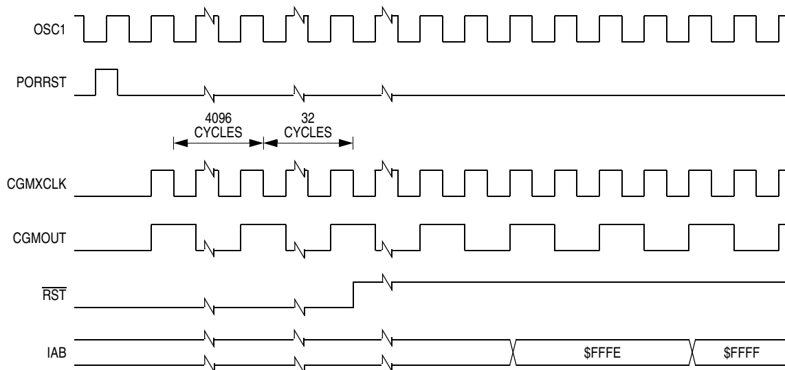
Figure 16-7. POR Recovery
