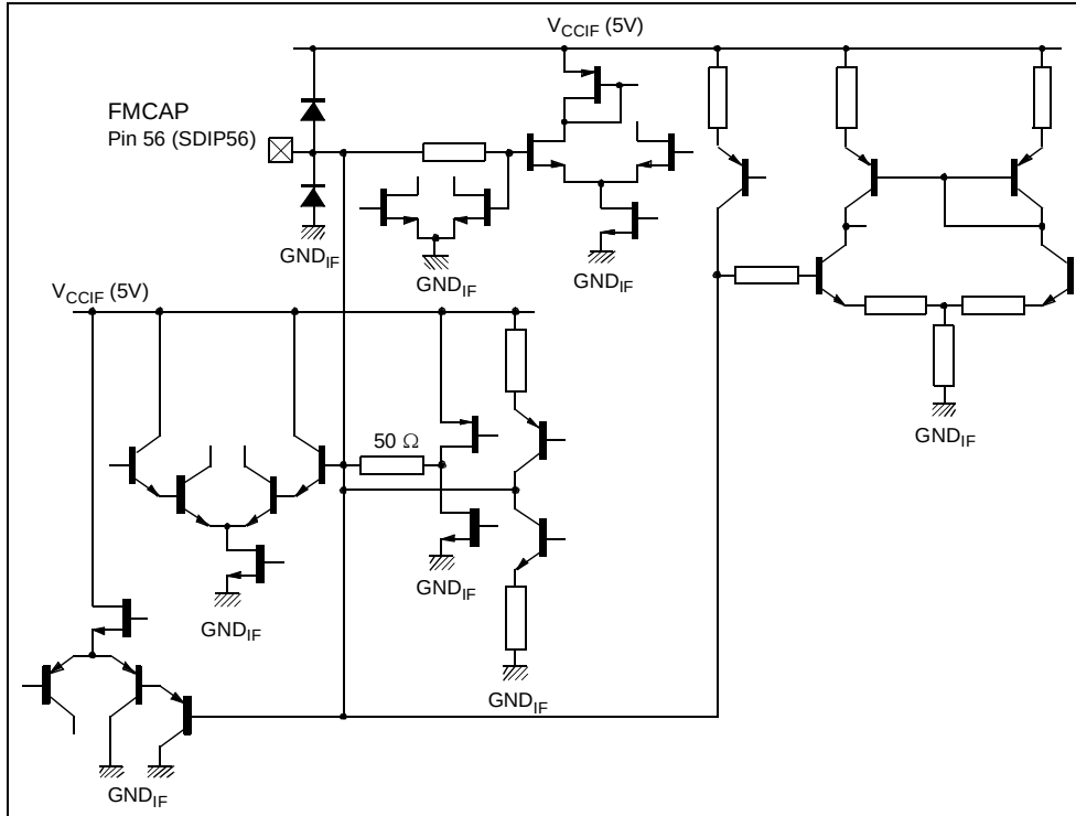
Figure 26. IF Inputs
