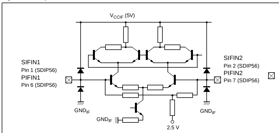
Figure 26. IF Inputs
