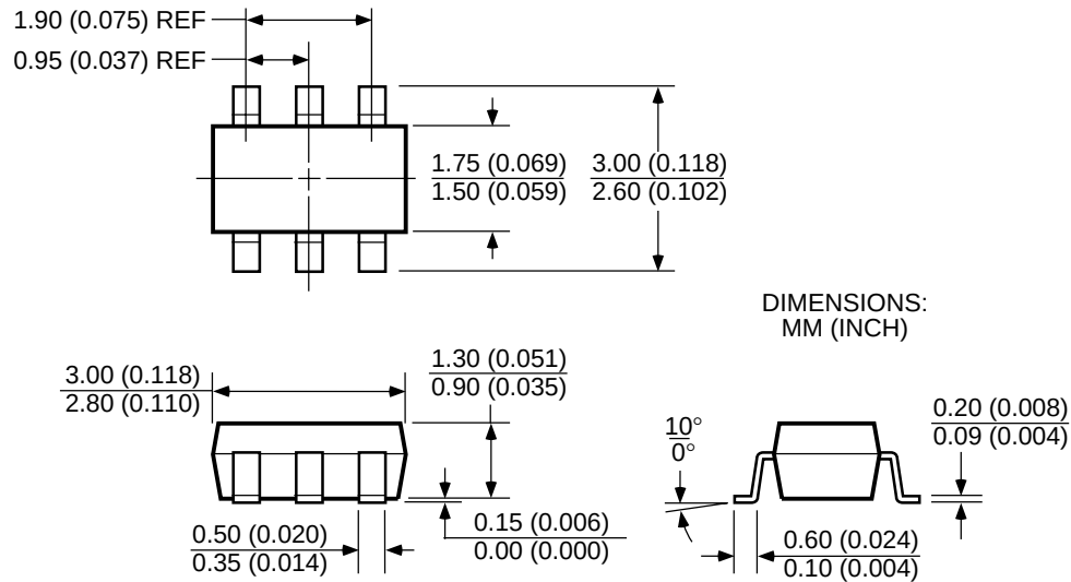
SOT-23-6 (M6)
