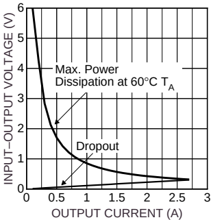
Si3445DV SOA
