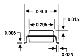
20-Pin SOIC Package
