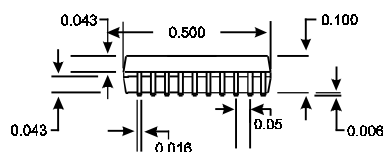
20-Pin SOIC Package
