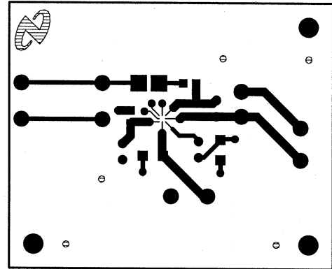
Top Layer
