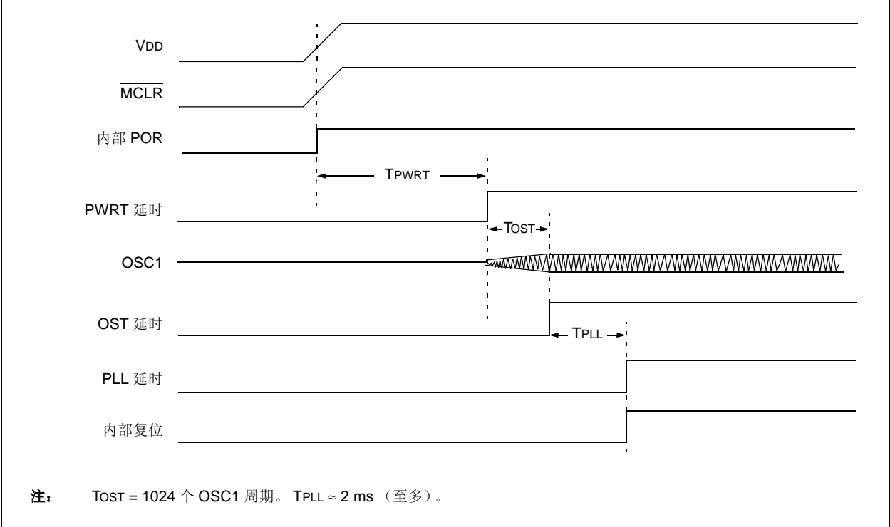
图 4-7: 在 PLL 使能时 POR 的延时时序 (MCLR 连接到 VDD)
