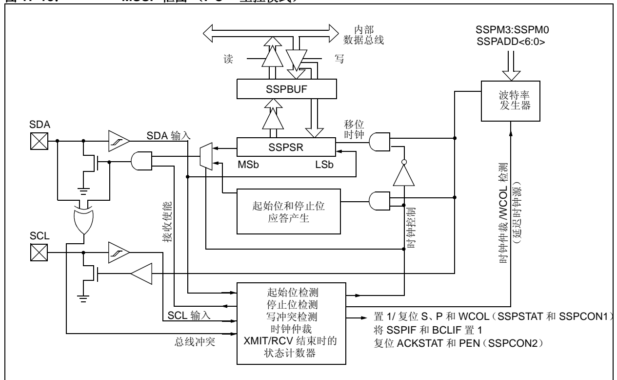
图 17-18: MSSP 框图 (I 2 C™ 主机模式)
