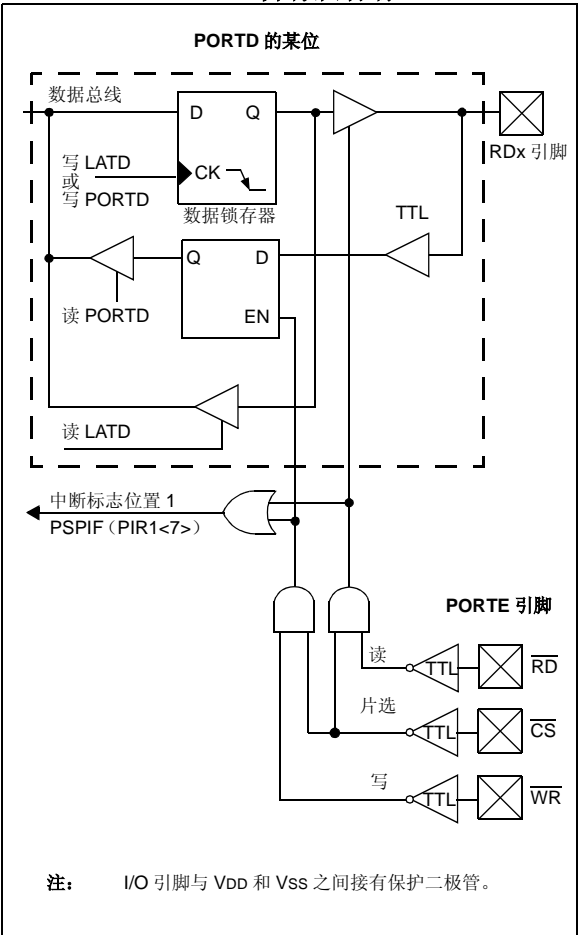
图 10-2: PORTD 和 PORTE 框图（并行从动端口）
