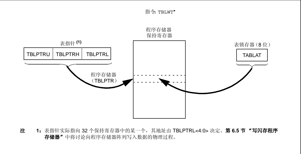
图 6-2: 表写操作
