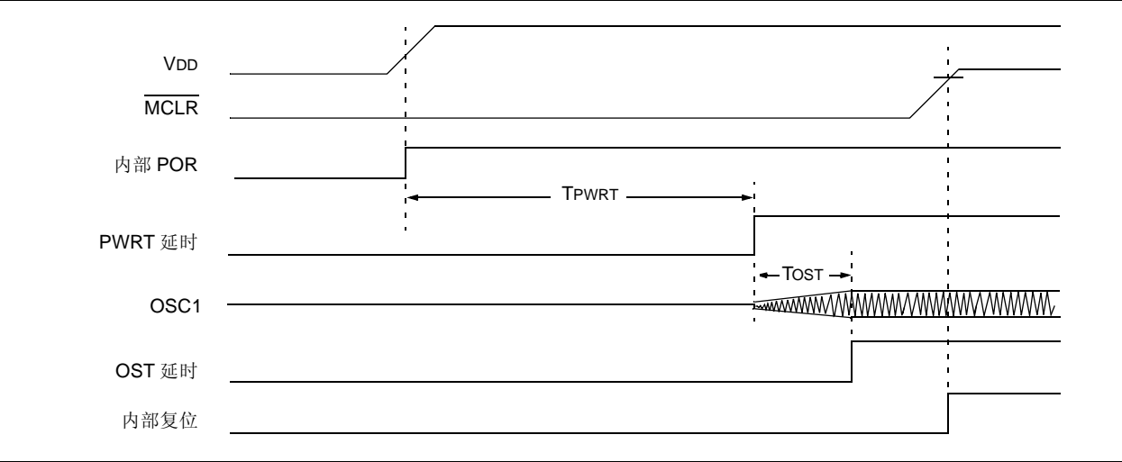
图 4-5: 上电延时时序 (MCLR 在 Tost 结束之后上升)
