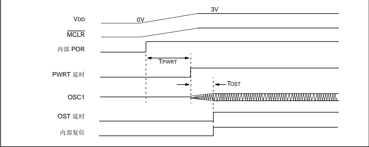
图 4-6: 缓慢 VDD 上升时间 (MCLR 连接到 VDD, VDD 电压上升时间 > TPWRT)
