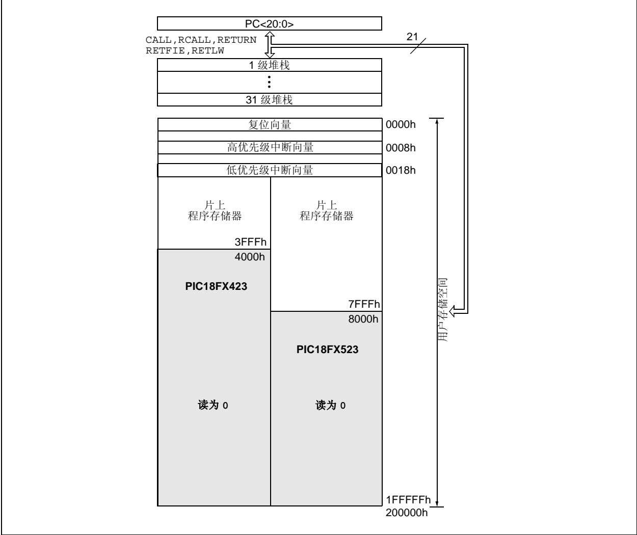
图 5-1: PIC18F2423/2523/4423/4523 器件的程序存储器映射和堆栈
