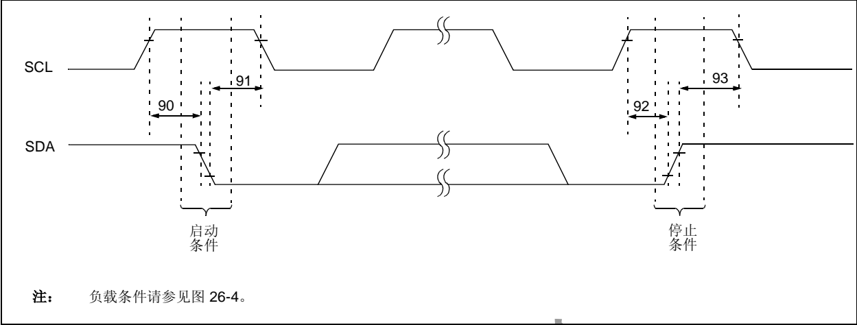
图 26-18: 主 SSP I 2 C™ 总线启动 / 停止位时序波形图
