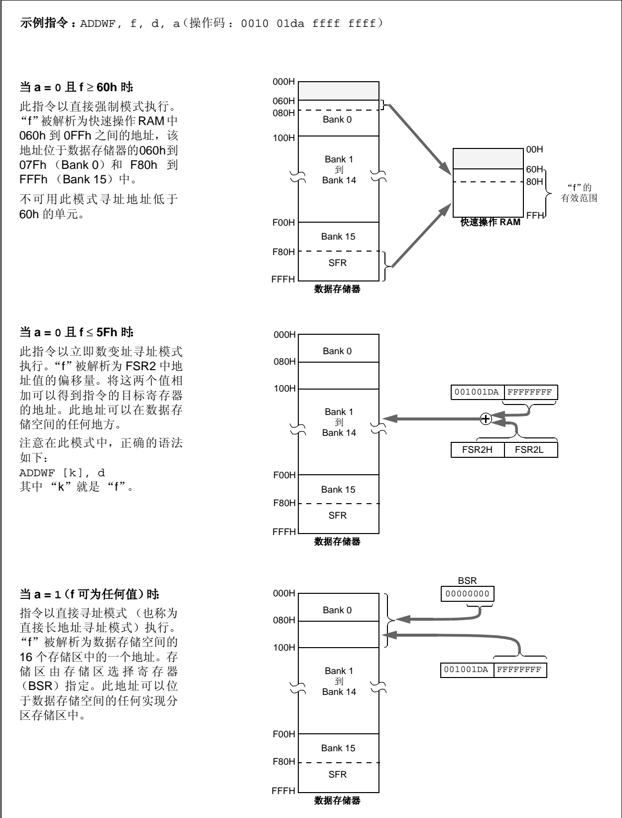
图 5-9： 针对位和针对字节的指令的寻址模式对比（使能了扩展指令集）
