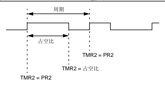
图 15-4: PWM 输出
