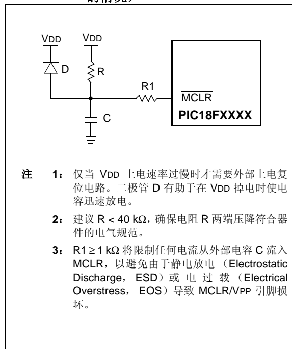
图 4-2：外部上电复位电路（ V_{DD} 缓慢上电的情况）
