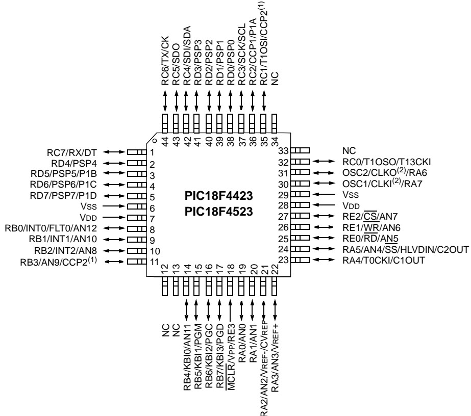
44 引脚 TQFP
