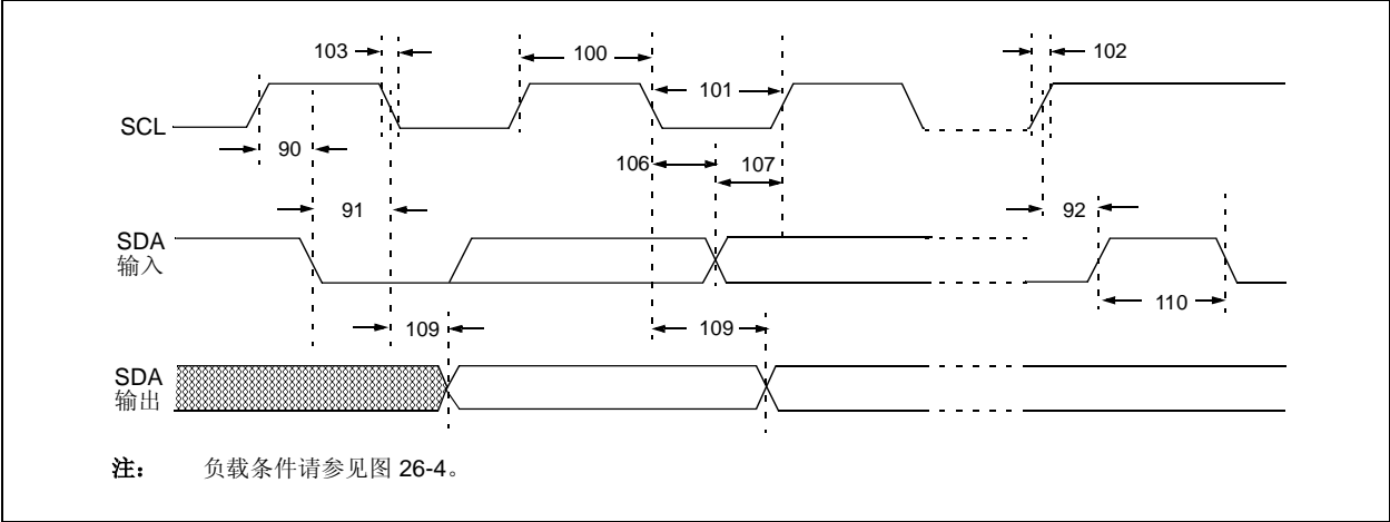
图 26-17: I 2 C™ 总线数据时序
