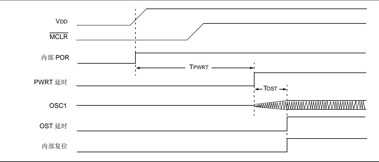
图 4-4: 上电延时时序 (MCLR 在 Tost 结束之前上升)
