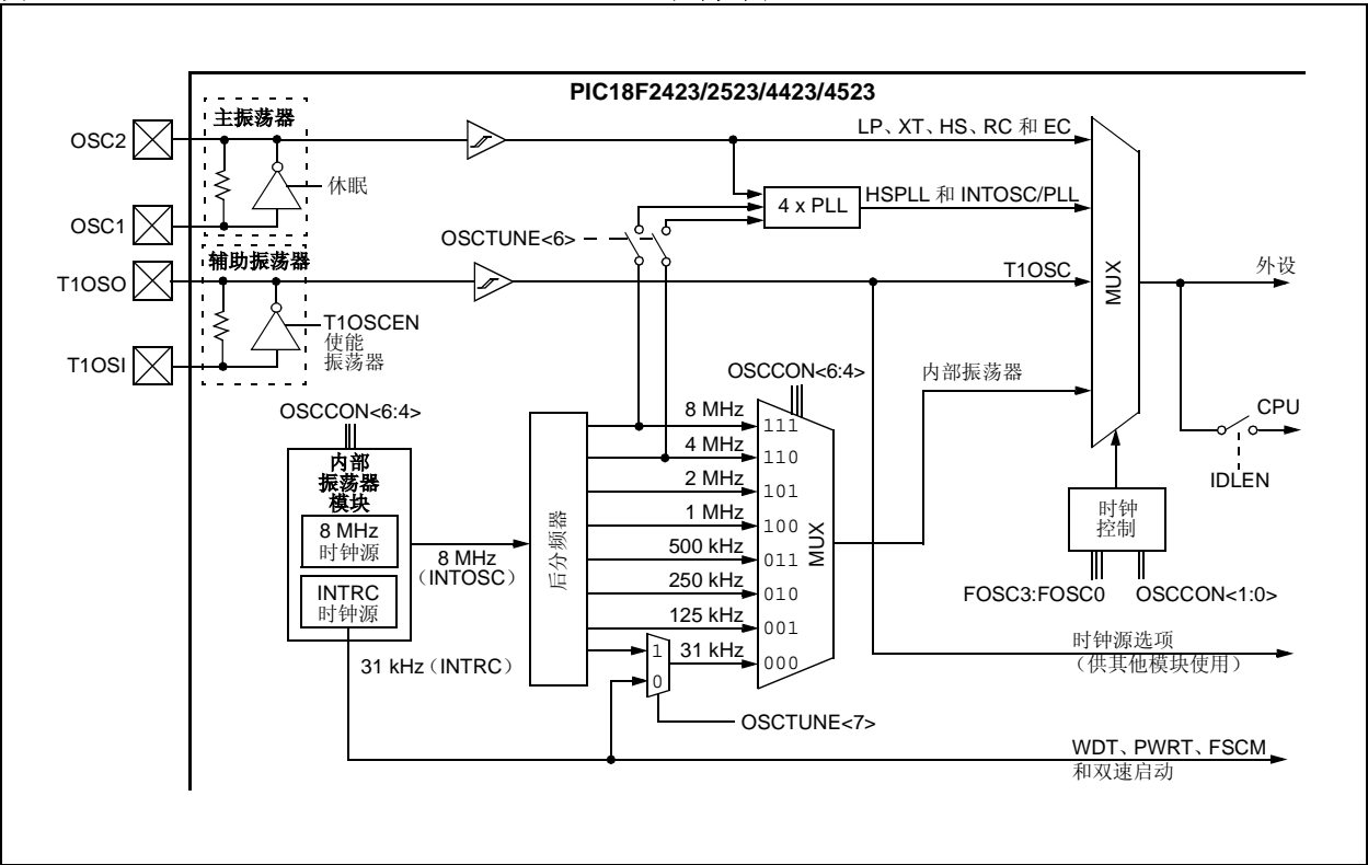
图 2-8: PIC18F2423/2523/4423/4523 时钟框图
