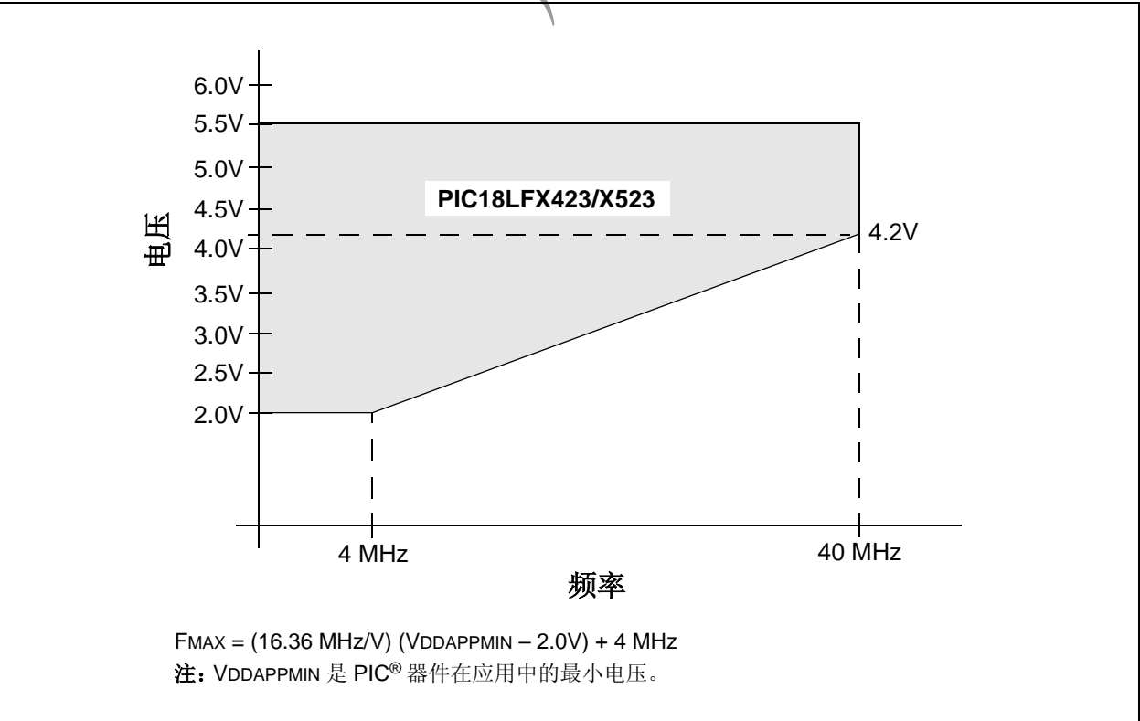
图 26-2: PIC18LF2423/2523/4423/4523 电压—频率关系图（工业级）
