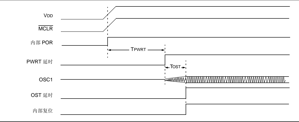
图 4-3: 上电延时时序 (MCLR 连接到 VDD, VDD 电压上升时间 < TPWRT)
