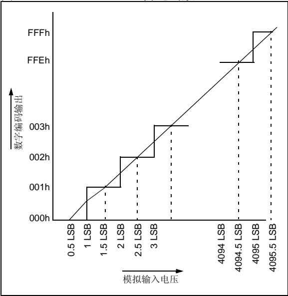
图 19-2: A/D 传递函数
