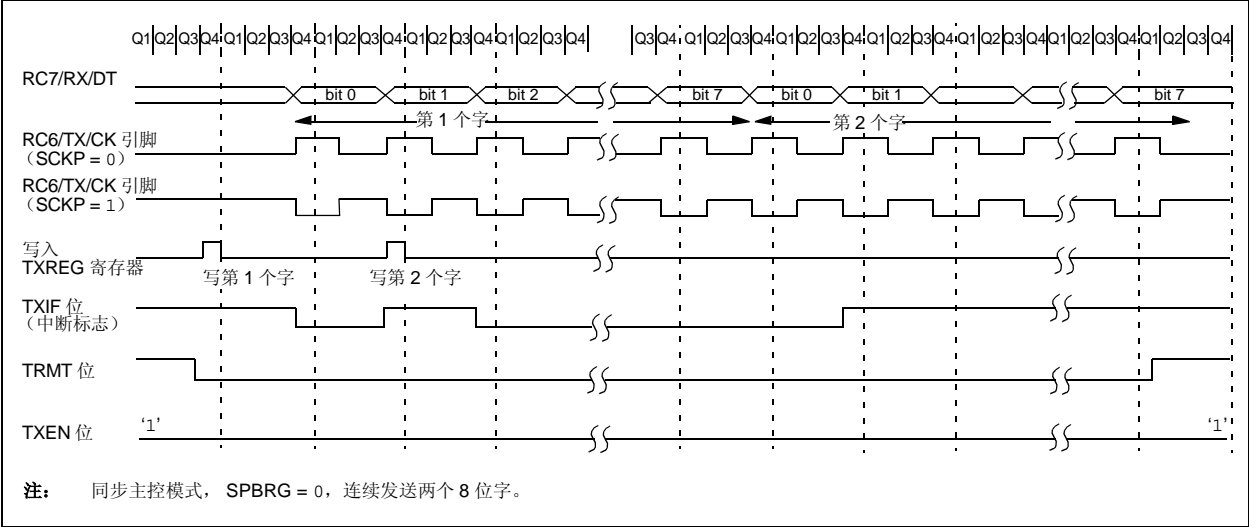
图 18-11: 同步发送
