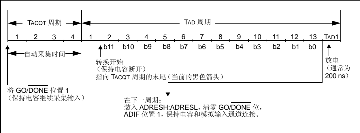
图 19-5: A/D 转换 TAD 周期 ( \text{ACQT}\langle 2:0 \rangle = 010 , \text{TACQ} = 4 \text{ TAD} )
