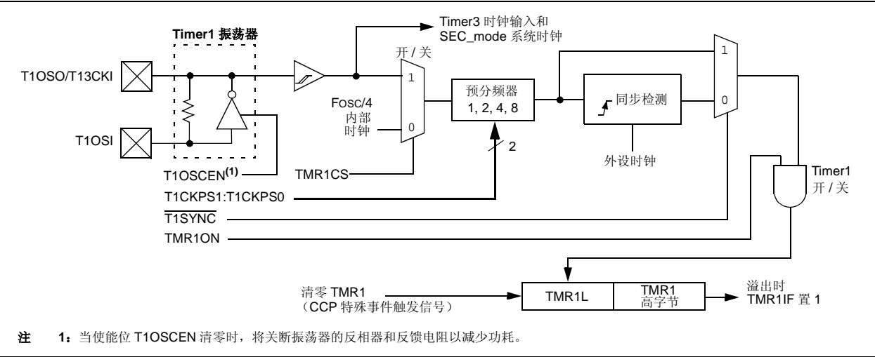
图 12-1: TIMER1 框图
