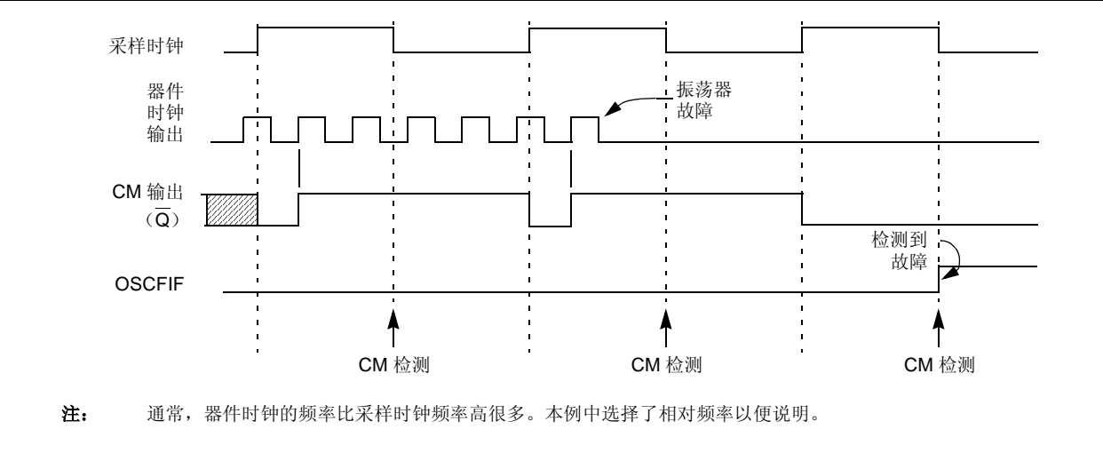
图 23-4: FSCM 时序图
