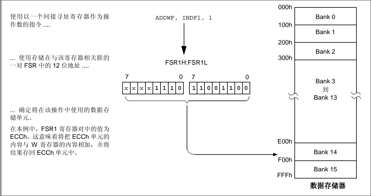
图 5-8：间接寻址
