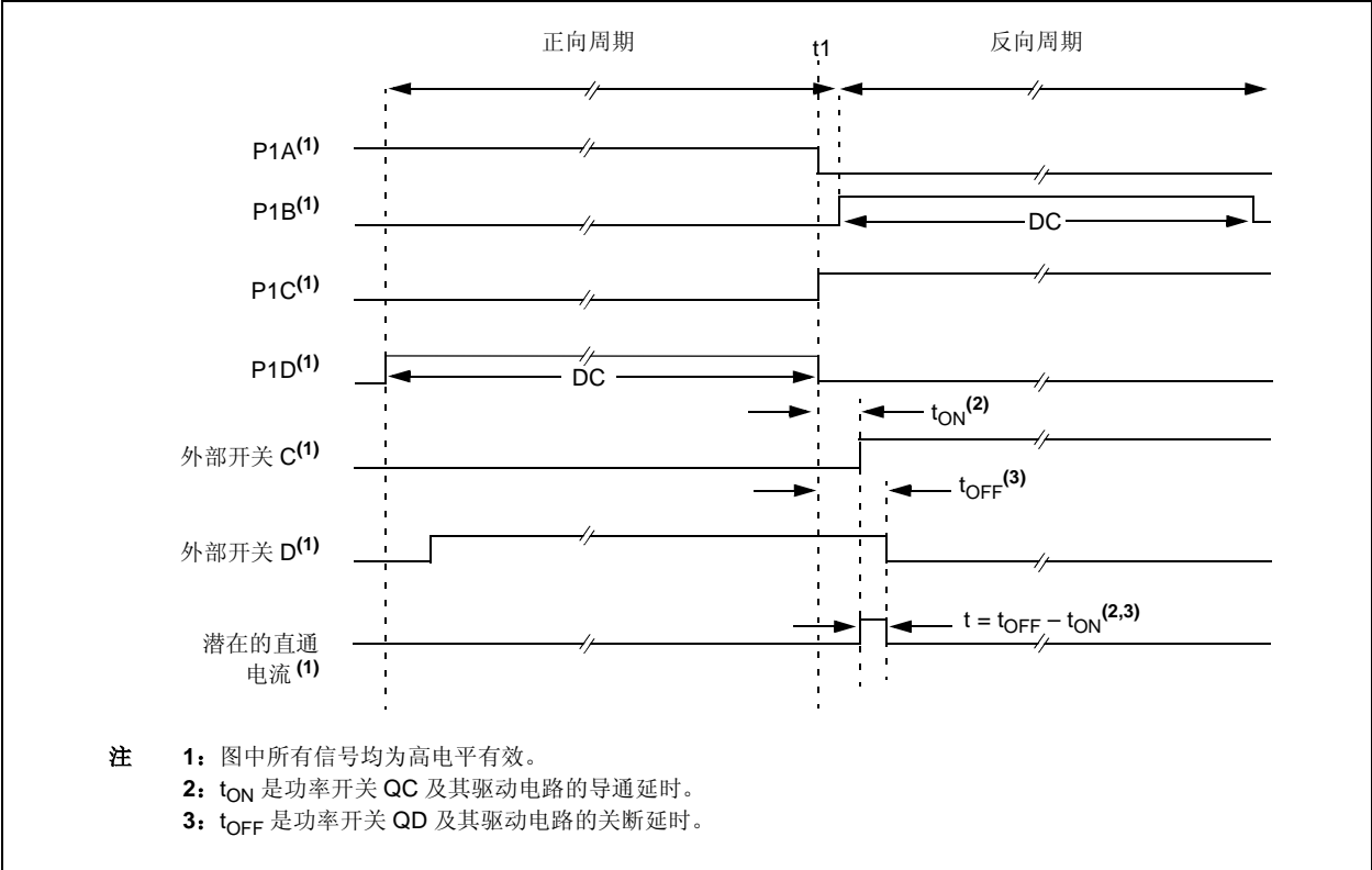
图 16-9: 在占空比接近 100% 时改变 PWM 方向
