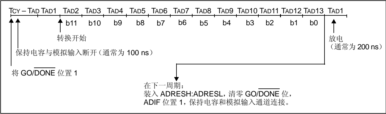
图 19-4: A/D 转换 TAD 周期 ( \text{ACQT}\langle 2:0 \rangle = 000 , \text{TACQ} = 0 )
