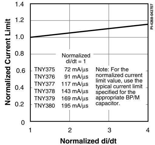
图 24. 限流点与 di/dt 的特性曲线
