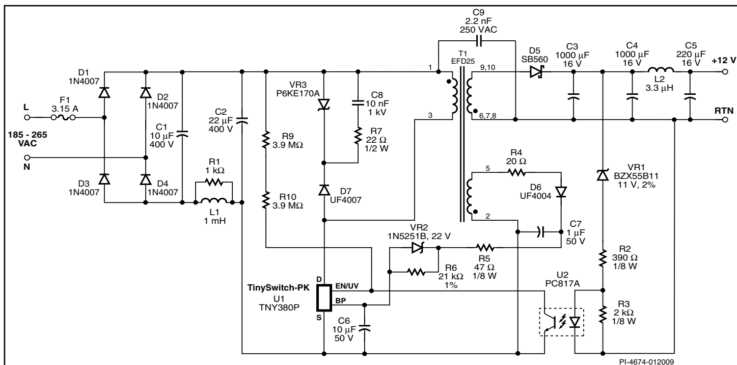
图 15. 使用 TNY380P 的通用电压输出、20 W 连续输入功率、45 W 峰值功率的电源
