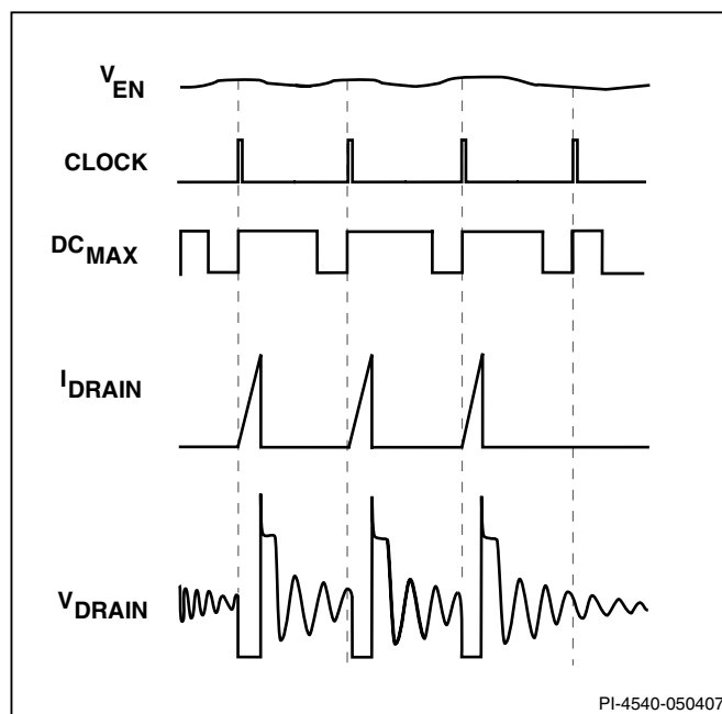
图 8. 在中等负载时的操作( f_{osc} 132 kHz)
