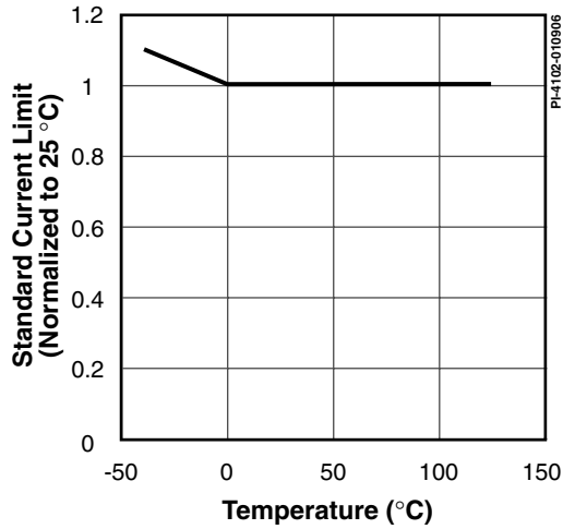
图 23. 标准限流点与温度的特性曲线
