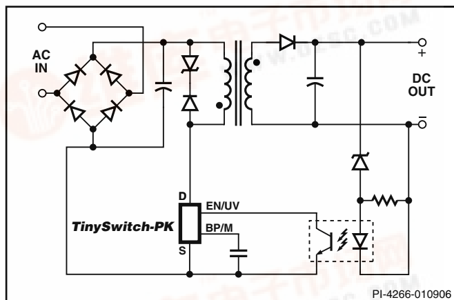
图 1. 典型峰值功率的应用
