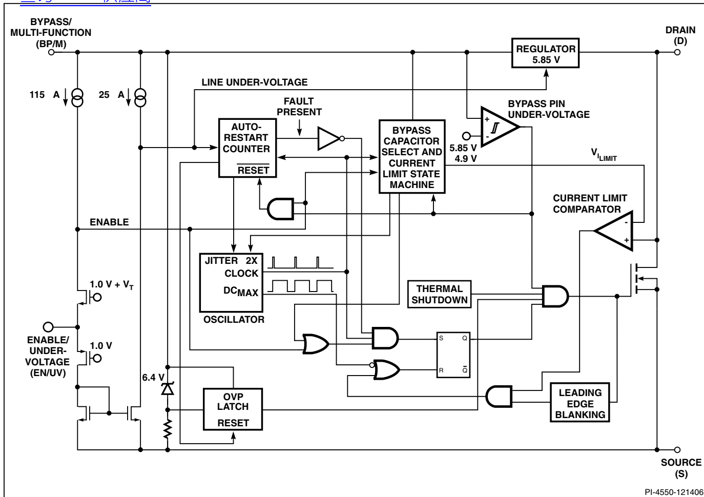
图2. 功能结构图
