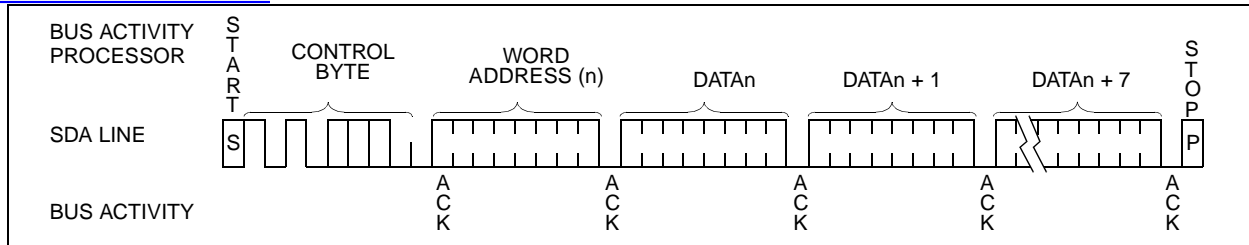
查询PIC16CE62X供应信息 FIGURE 6-6: PAGE WRITE
