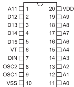
HT604L — 20 DIP-B/SOP-A
