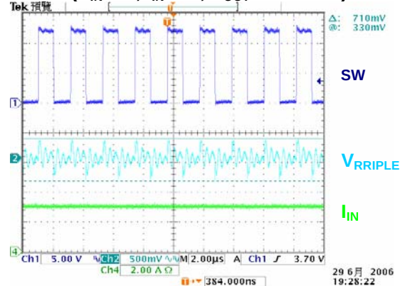
VOUT RIPPLE=710mV ( V_{IN}=6V , I_{IN}=3A , V_{OUT}=12V/1.4A )
