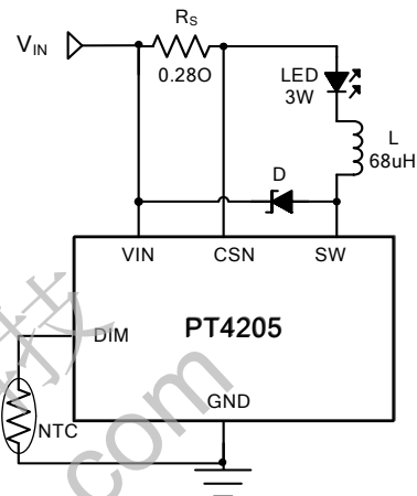
利用 NTC 实现 LED 工作温度补偿
