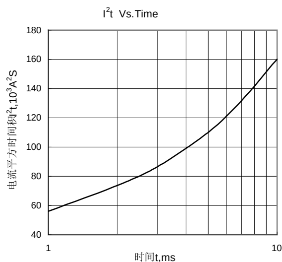
Fig.3 I^2t 特性曲线
