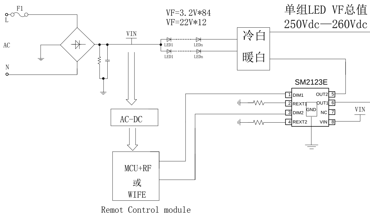
图2 SM2123E 智能冷暖双色恒功率系统
