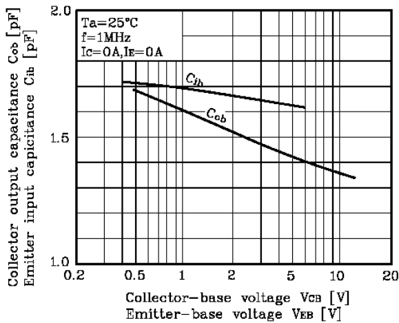
Fig. 5 C_{ob}-V_{CB} , C_{ib}-V_{EB}
