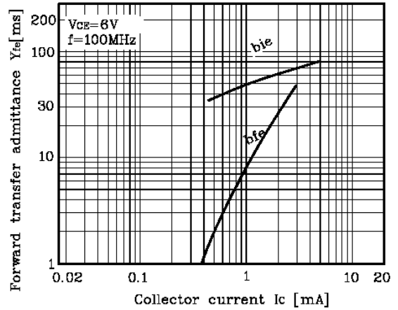
Fig. 8 I_C - Y_{fe}
