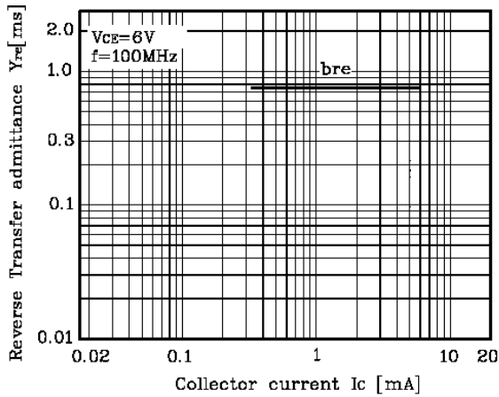
Fig. 9 I_C - Y_{re}
