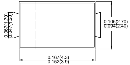
SMA/DO-214AC
