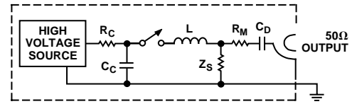
Figure 21. EFT Generator
