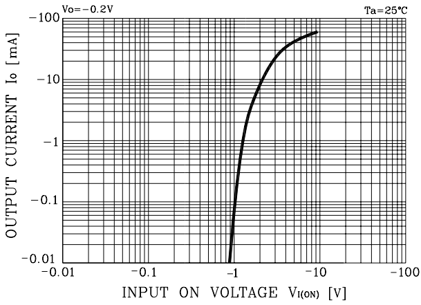
Fig. 3 G_1 - I_o
