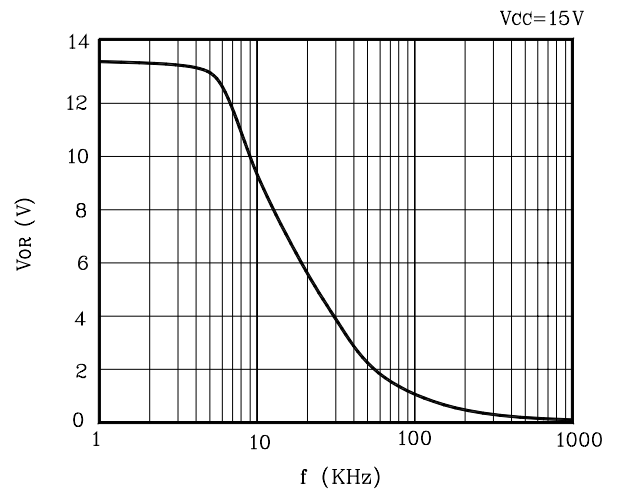
Fig. 4 V_{OR}-f
