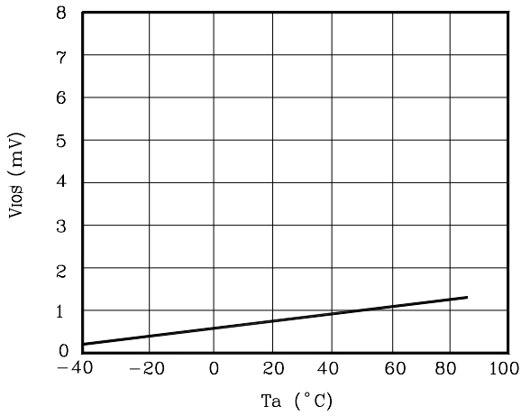
Fig. 1 V_{Ios}-T_a
