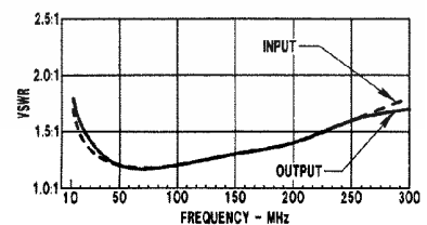
Input/Output VSWR
