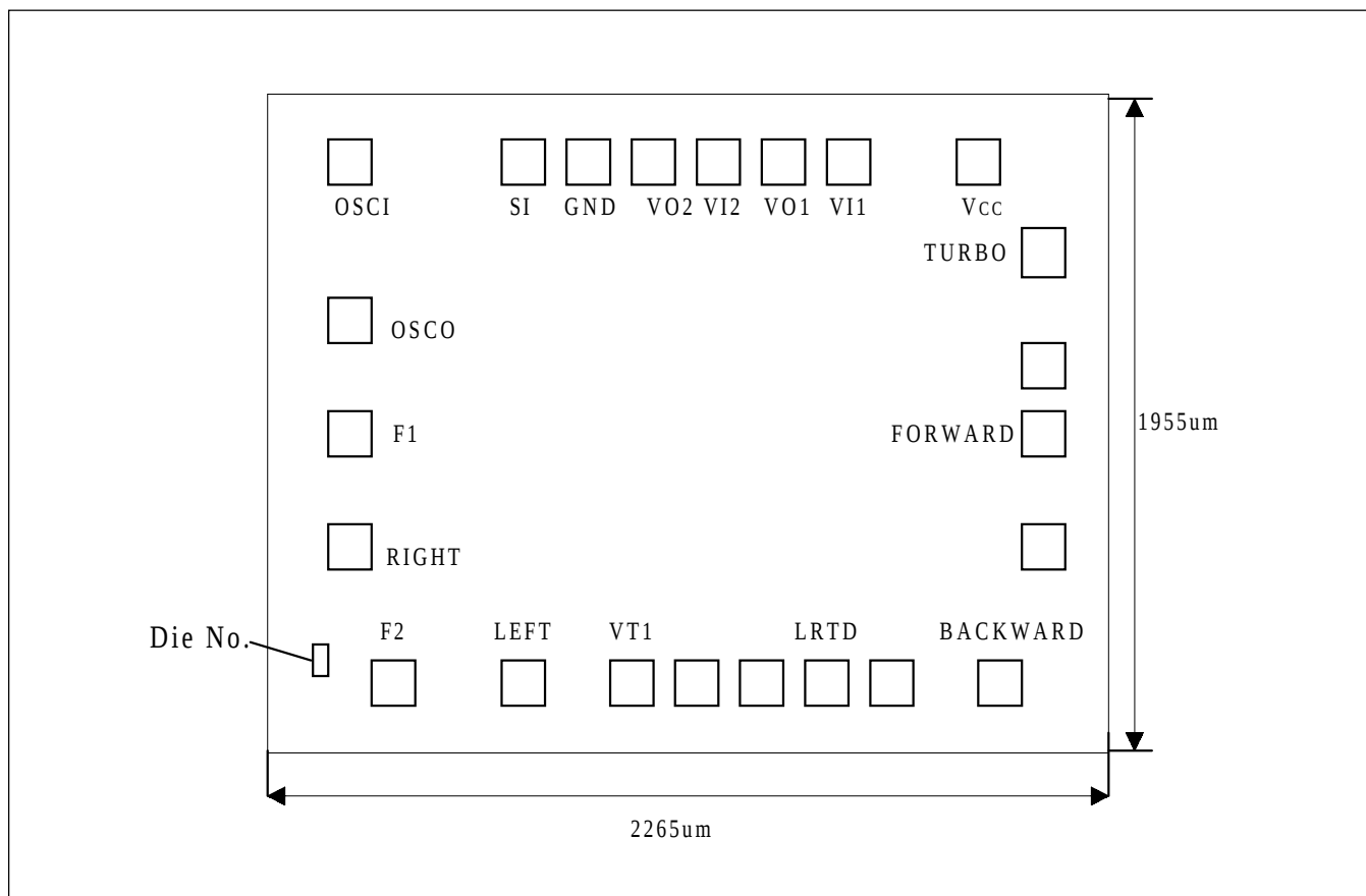
Pad Coordinates
