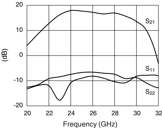
S-Parameters
