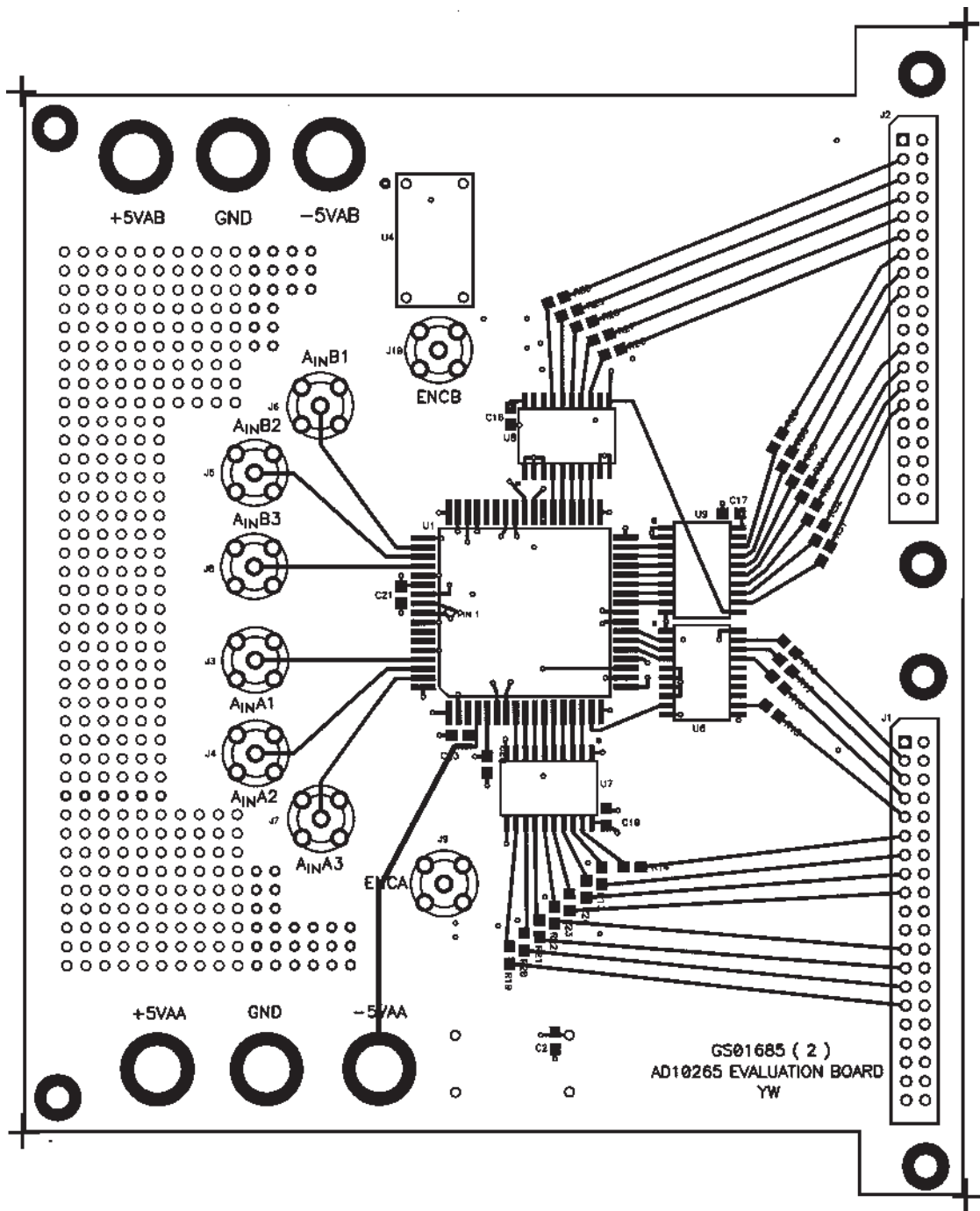
Figure 23. Top Layer
