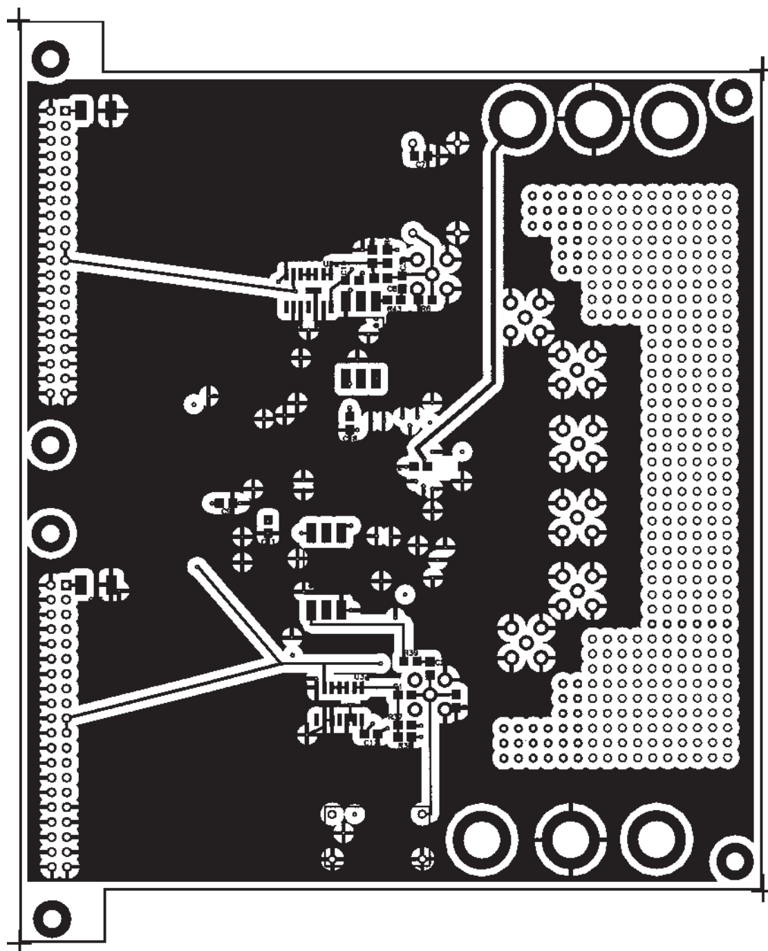
Figure 24. Bottom Layer
