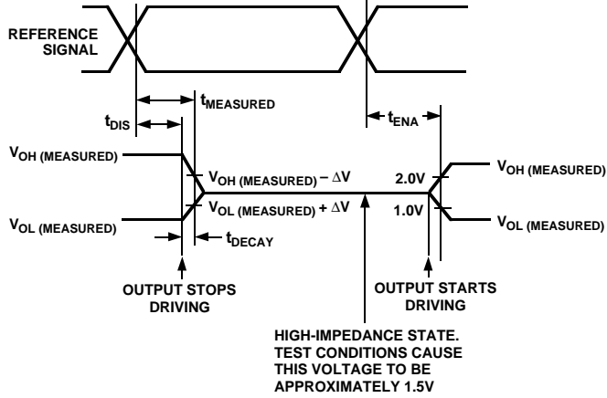
Figure 27. Output Enable/Disable
