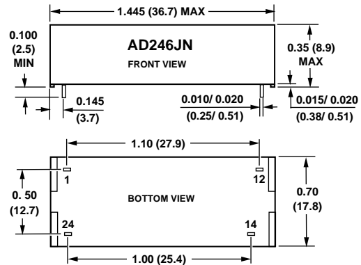
AD246JN Package
