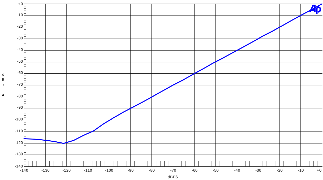
Linearity(fin=1kHz)
