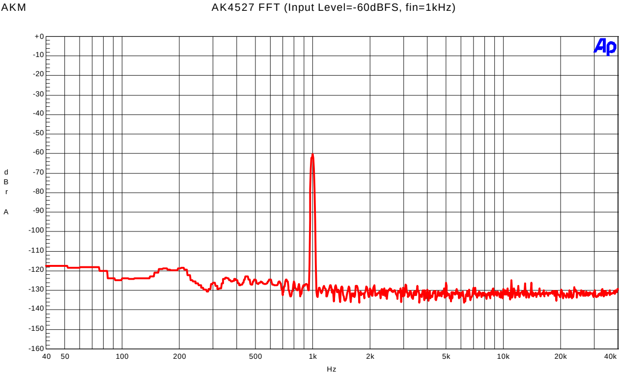
FFT (Input=-60dBFS,fin=1kHz)
