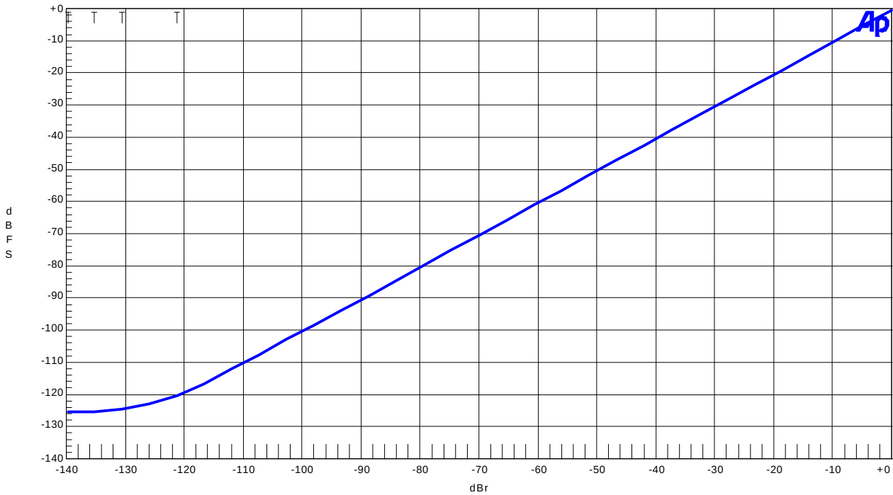
Linearity(fin=1kHz)
