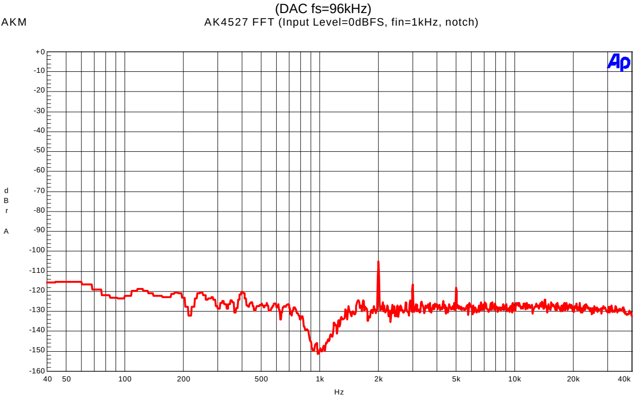
FFT (Input=0dBFS, fin=1kHz, Notch)
