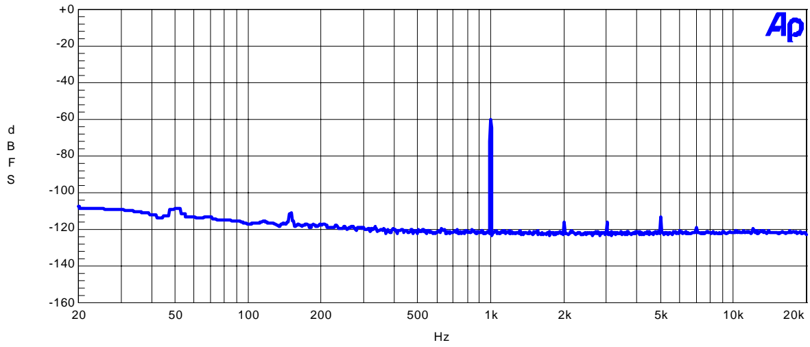
Fig7.FFTPlot
