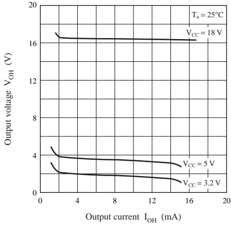
V_{OH} - I_{OH}
