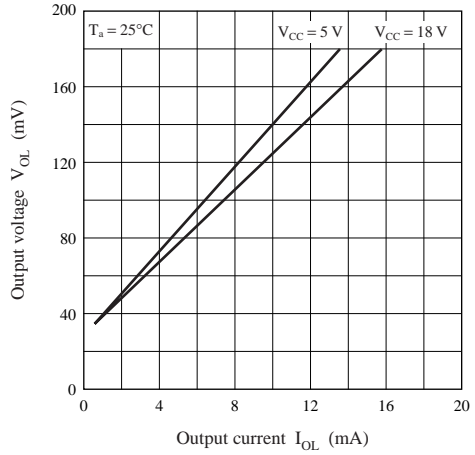
V_{OL} - I_{OL}
