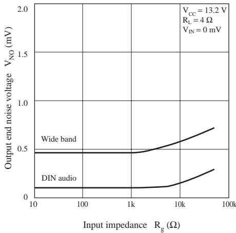
V_{NO} - R_g
