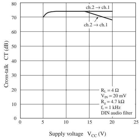
CT — V_{CC}
