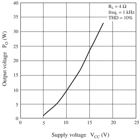
P_O - V_{CC}
