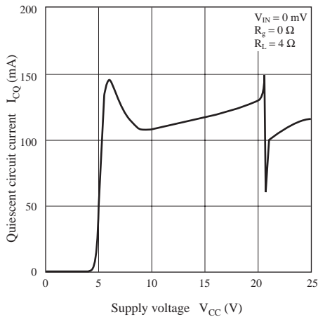
I_{CQ} — V_{CC}
