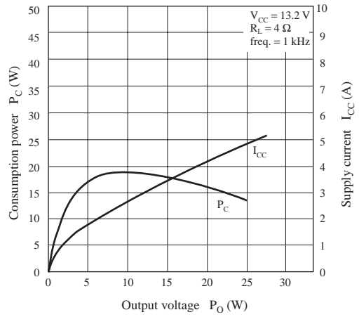
P_C, I_{CC} - P_O
