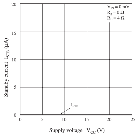
I_{STB} — V_{CC}
