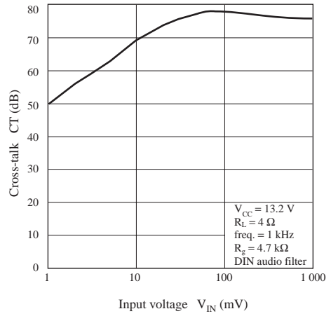
CT — V_{IN}
