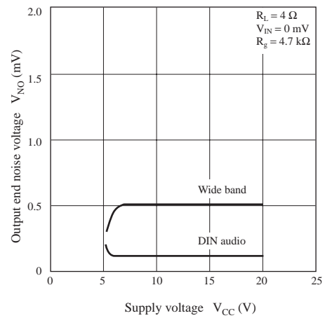
V_{NO} - V_{CC}
