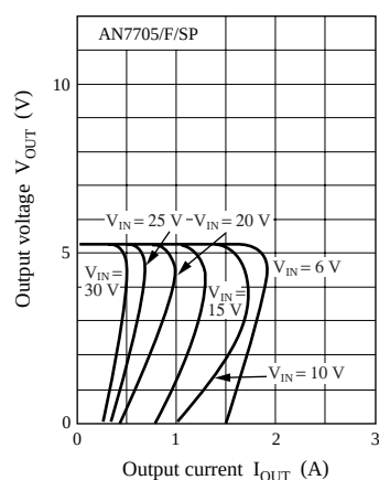
V_{OUT} - I_{OUT}
