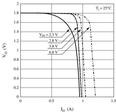
V_O - I_O
