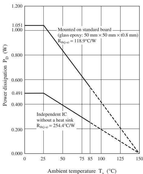
P_D — T_a
