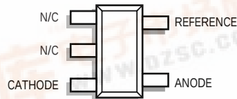
SOT-23/5L (DBV)
