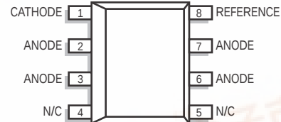
SOIC (D)
