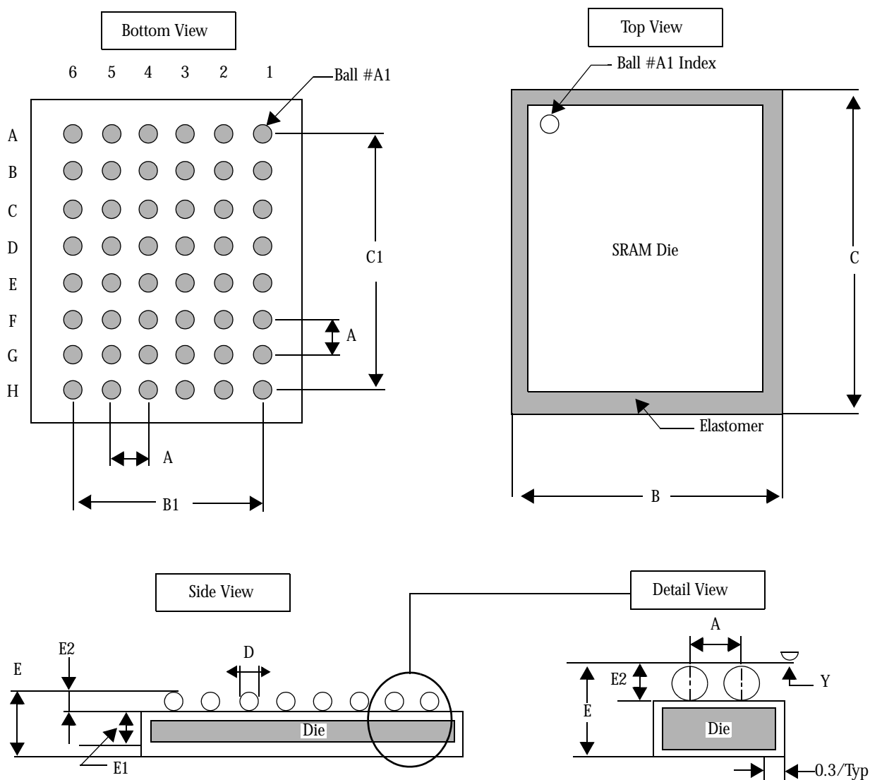
48-ball FBGA
