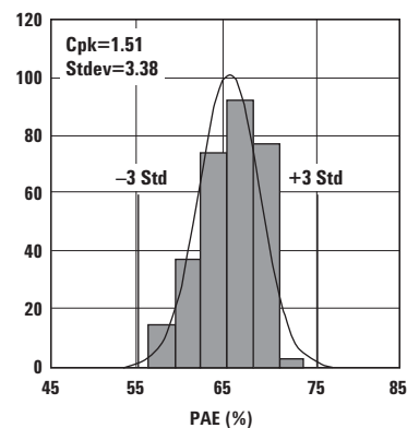
Figure 3. PAE.
