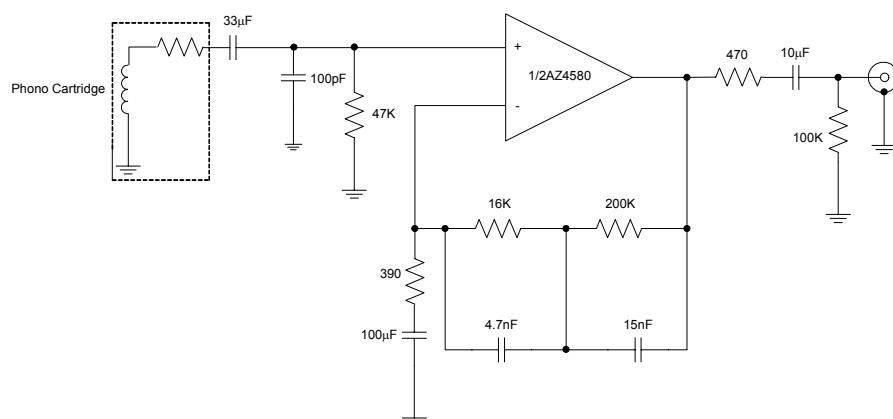
Figure11. RIAA Preamp
