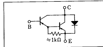
内部接続図 / Connection Diagram
