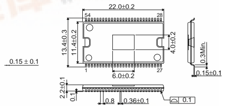
SSOP-A54
