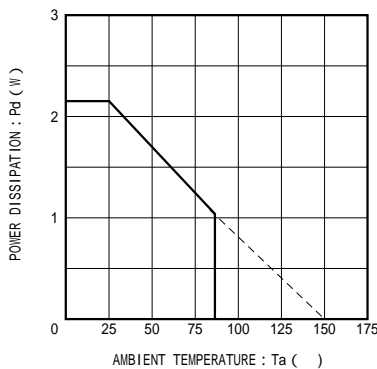
Fig. 3 熱軽減曲線
