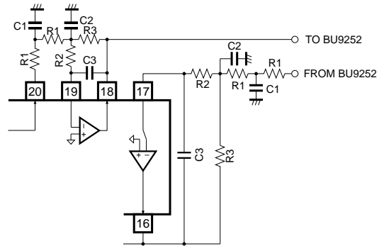
Fig. 4 LPF
