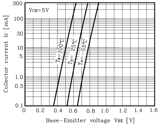
Fig. 2 I_C - V_{BE}
