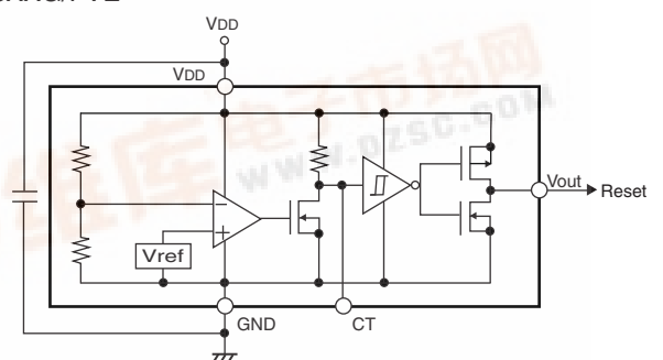
BD53XXG/FVE
