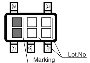
BD52XXFVE/BD53XXFVE : VSO5 (EMP5)
