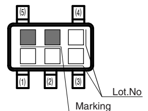
BD52XXFVE/BD53XXFVE : VSO5 (EMP5)
