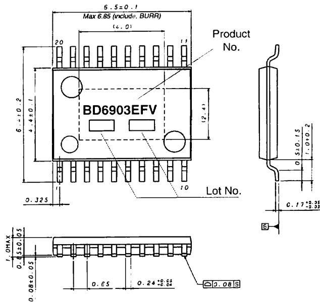
HTSSOP-B20 (Unit:mm)
