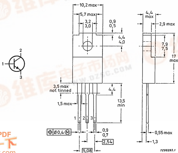
Fig.1 SOT186.
