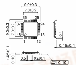
VQFP48
