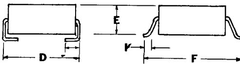
DO-214AA
